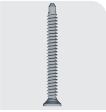
Schraube mit Vollge- winde ST6,3 x 60 (T25)
